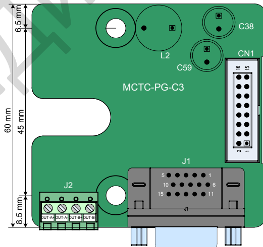
Рис. 3-30 MCTC-PG-C3 внешний вид и размеры (дифференциальный выход)
