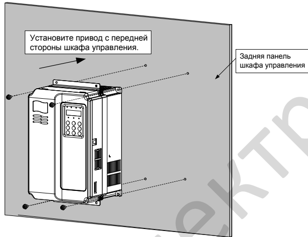
Рис. 3-2 Установка на заднюю панель ME320LN (пластиковый корпус)
