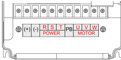
Рис 3-14 Расположение клемм силовой цепи (7.5–30 кВт)
