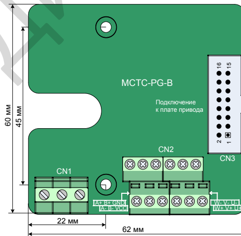
Рис. 3-27 MCTC-PG-B внешний вид и размеры
