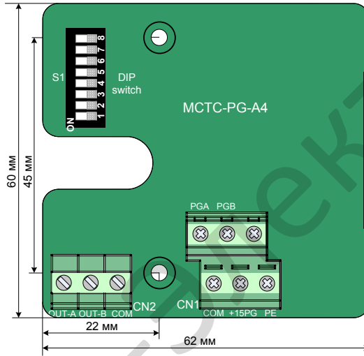
Рис. 3-25 МСТС-PG-A4 внешний вид и размеры
