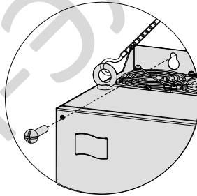
Рис. 3-7 Поднятие ME320LN (металлический корпус)
