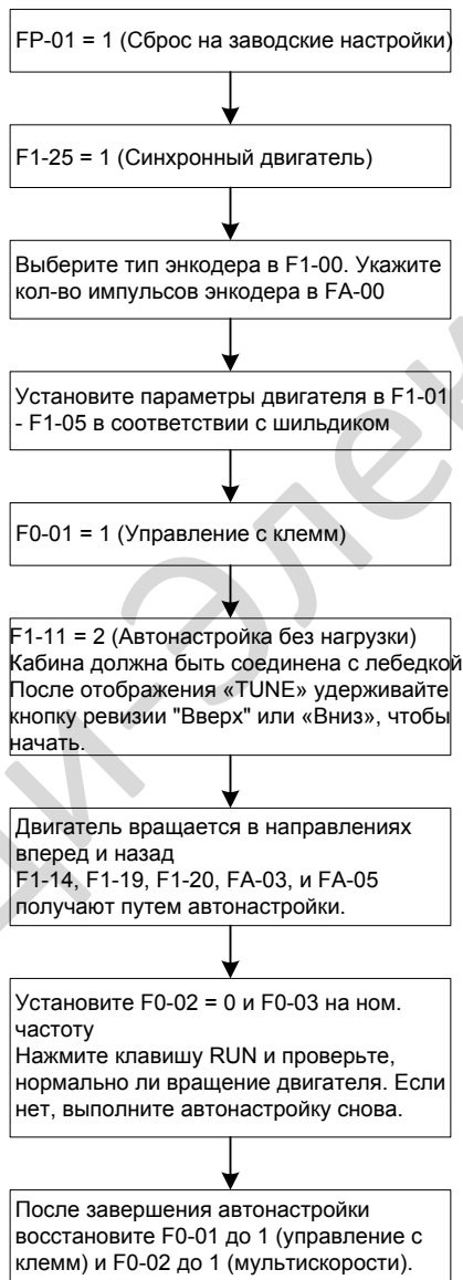
Рис. 7-3 Последовательность автонастройки без нагрузки синхронного двигателя
