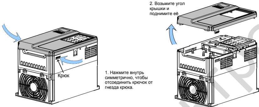
Рис. 3-12 Снятие передней крышки ME320LN (металлический корпус)
