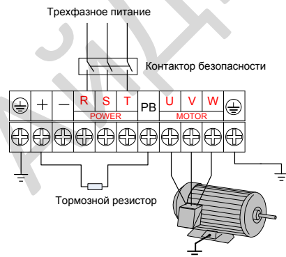
Рис 3-15 Диаграмма подключения силовой цепи
