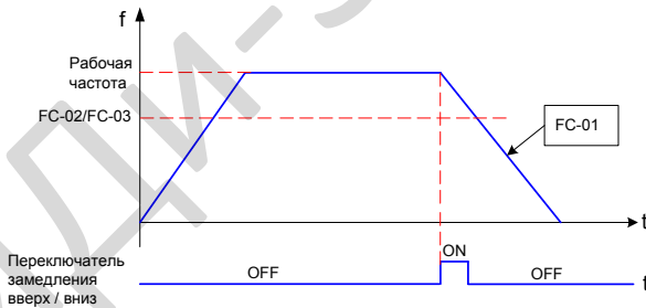
Рисунок 6-12 Принцип работы
