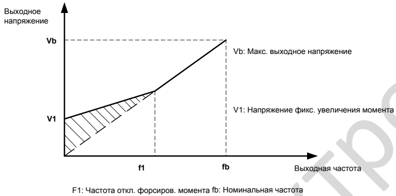
Рис. 6-15 Индивидуальное увеличение крутящего момента
