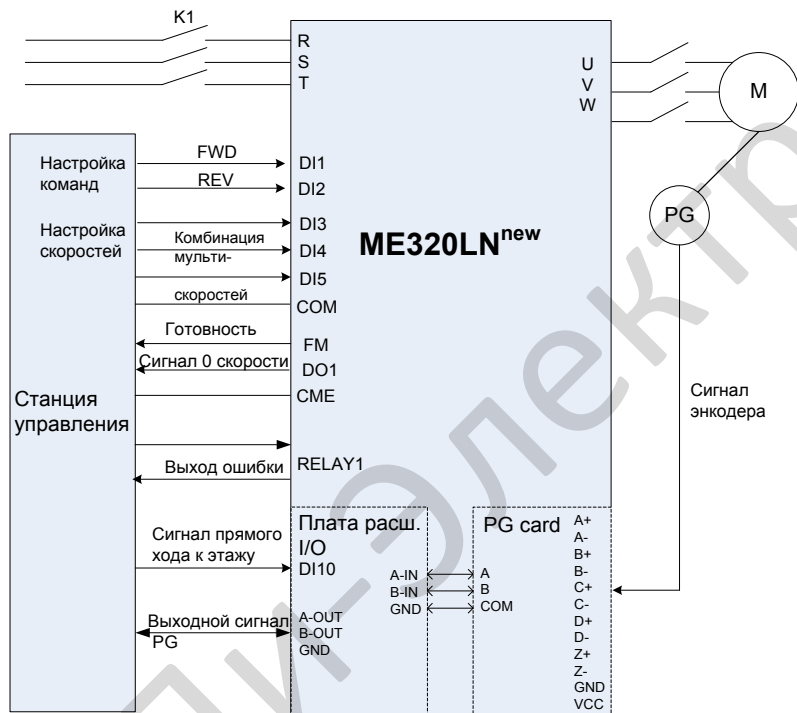
Рис. 7-13 подключение функции прямого хода к этажу
