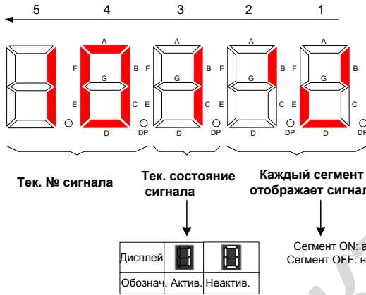
Рис 6-17 Пример состояния входов/выходов
